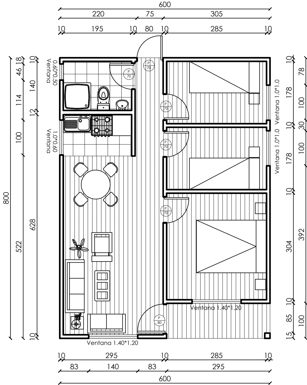
PLANTA ARQUITECTURA RUCALHUE 48 M2
